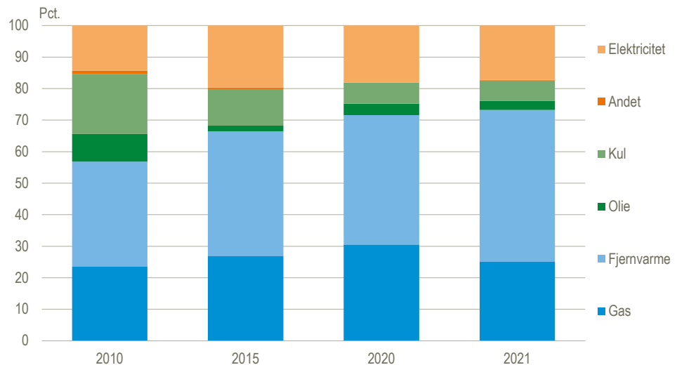
Figur 25 Energiforbrugets sammensætning i væksthushaverne
