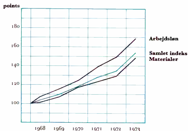
Byggeomkostningsindeks for et enfamiliehus 1968-73. 1. januar 1968 = 100
