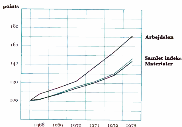
Byggeomkostningsindeks for en etageejendom, opført som montagebyggeri 1968-73. 1. januar 1968 = 100
