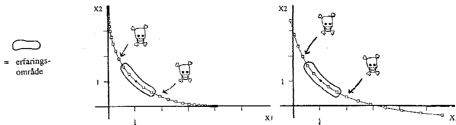
Figur 3. Isokvantdiagram, CES hhv. GL, \sigma = 2
