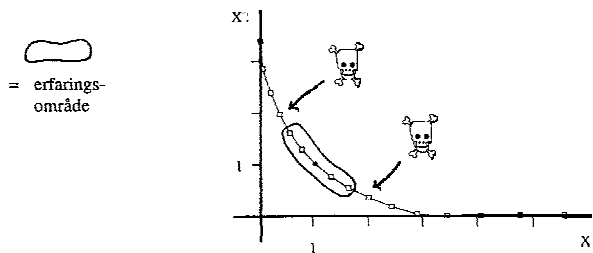
Figur 4. GL-isokvant med ikke-negativitetssikring
